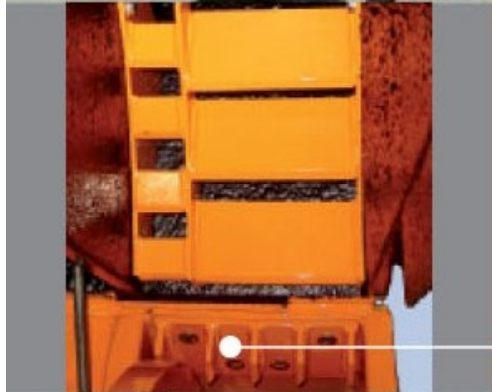
In der oberen Abdeckung montierter Zerhacker zur Nachzerkleinerung des Hackguts (Option)
