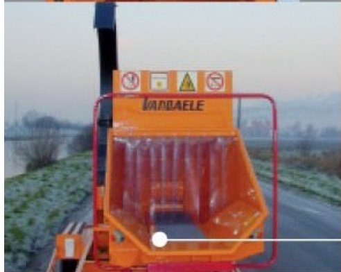
Trichter mit Gummi-Einfuhrband (Recycling-Unternehmen)
