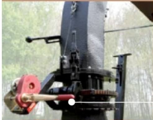
Nach unten klappbares Auswurfrohr (Option)
